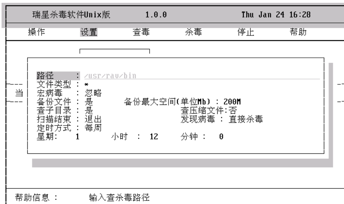
图 10 定时查杀设置界面
