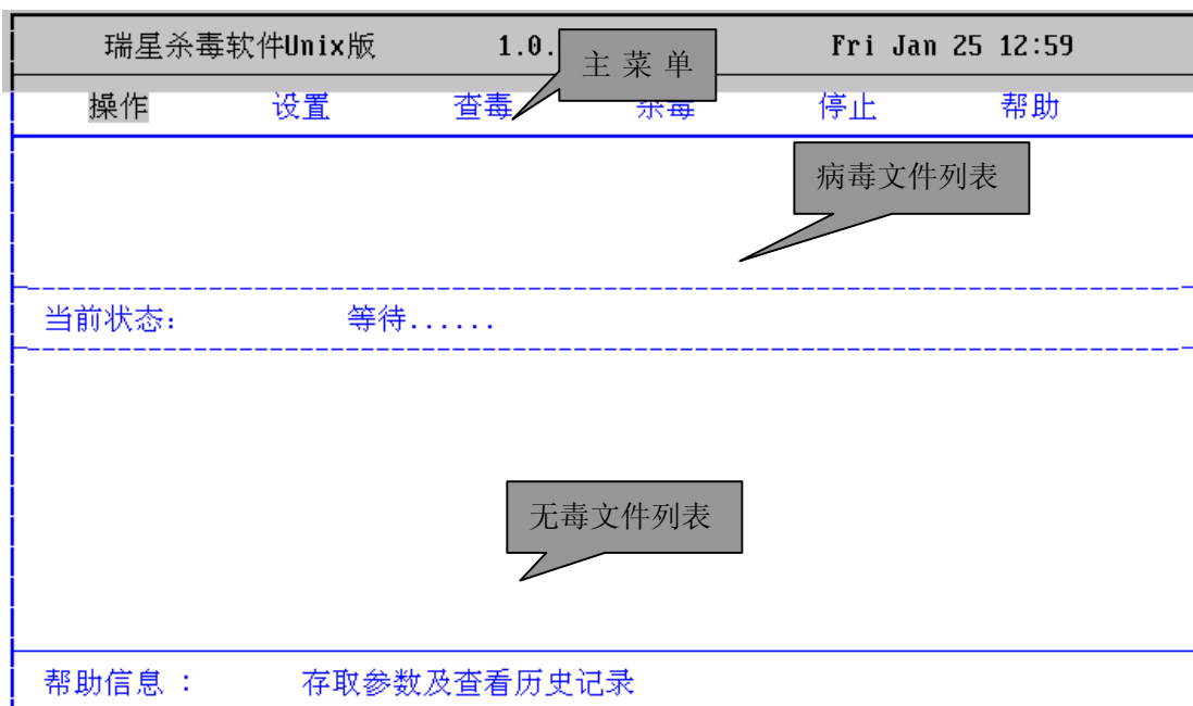
图 3 本地操作主界面
